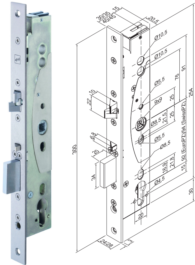
Abbildung und Masszeichnung zeigen die Rohrrahmenversion
