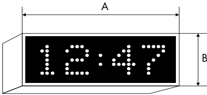
Montage apparent
